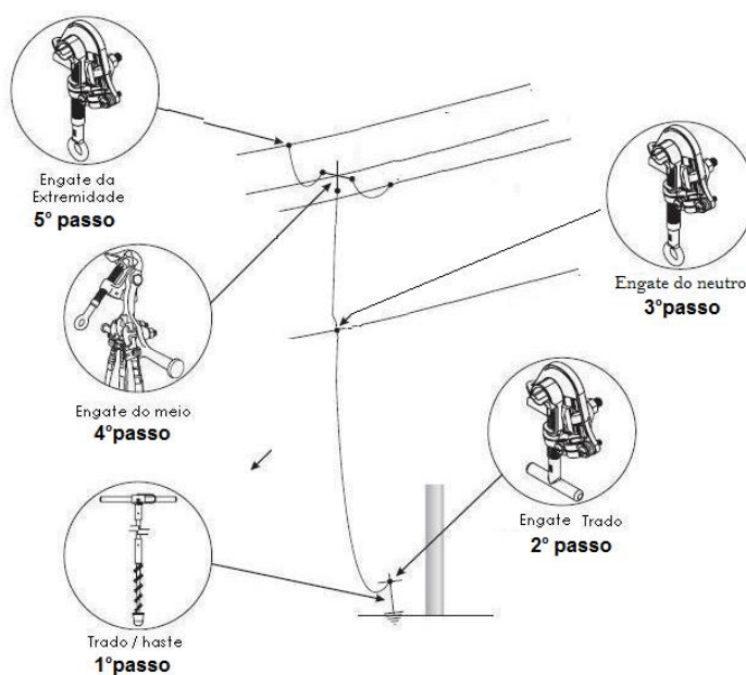
Figura 07 - Aterramento temporário de Média tensão
